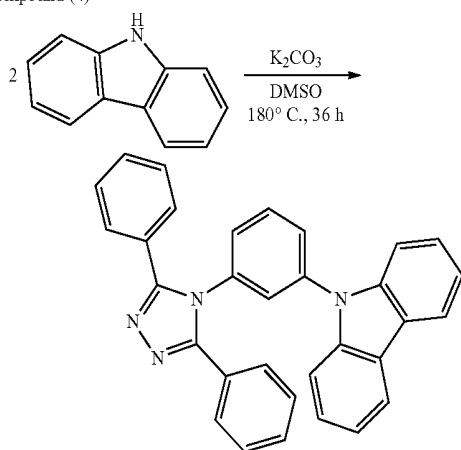
m-TAZCz
